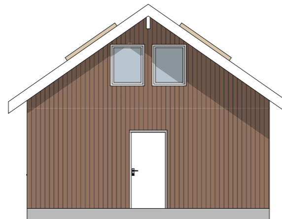
1:100 Fasade Sør
